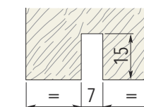
Detail vyfrézovaného dveřního křídla
